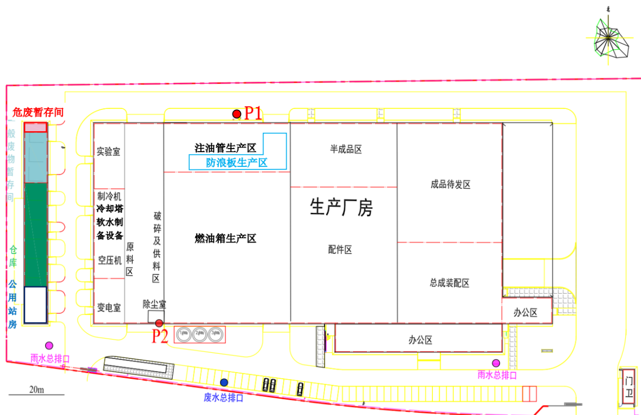
图 2.1-1 厂区平面布局图
