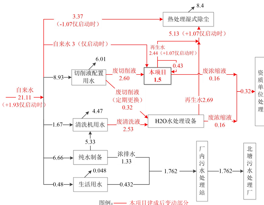
图 2.2-2 本项目建成后全厂水平衡图 (单位: m 3 /d)
