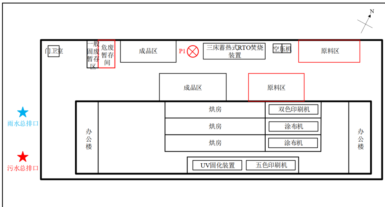
图 2.1-1 厂区平面布局图
