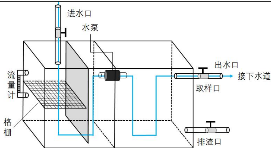
图 4 污水处理设备结构示意图
