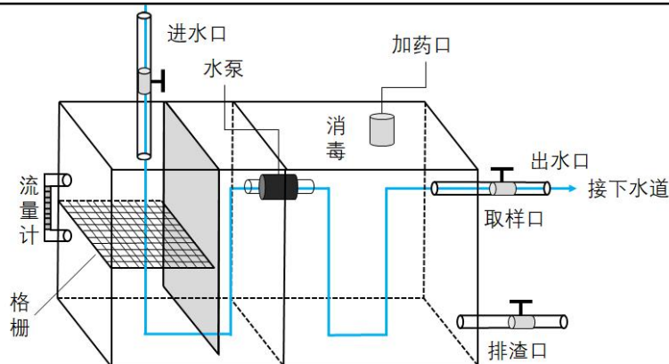
图 4 污水处理设备结构示意图
