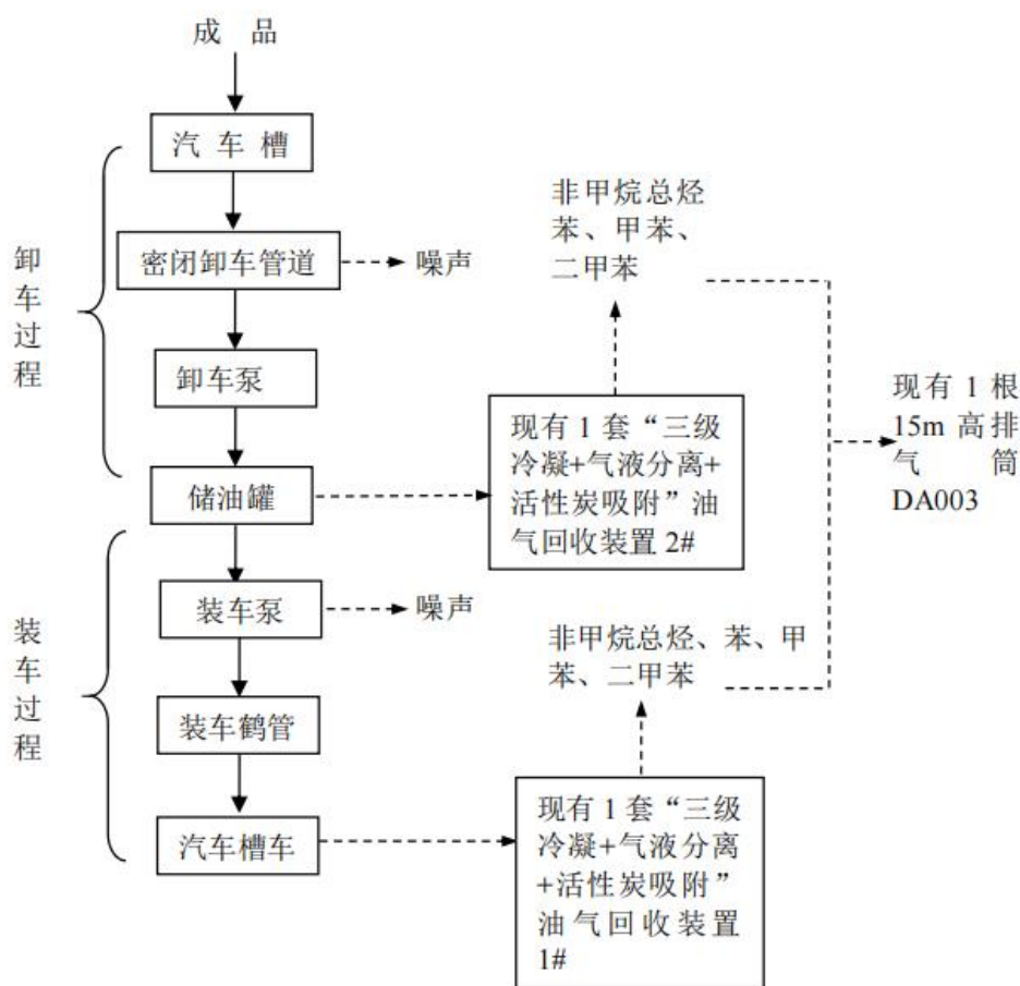
图 2-3 装卸车过程工艺流程图
