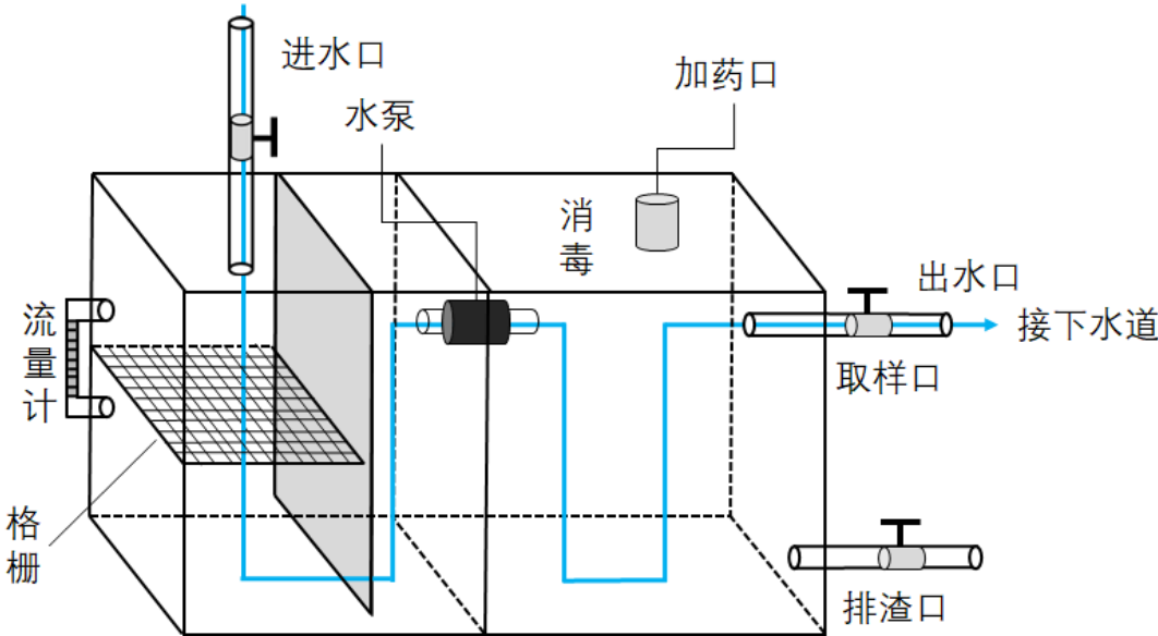
图 4-1 污水处理设备结构示意图
