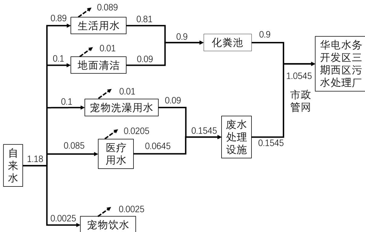
图 2-2 本项目水平衡图 单位 (m³/d)
